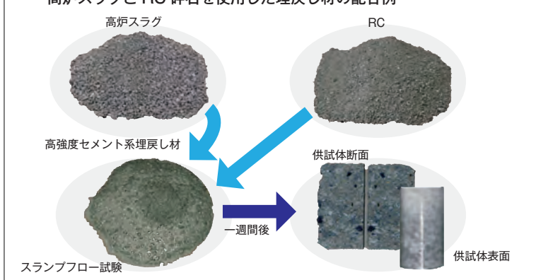
高炉スラグとRC 碎石を使用した埋戻し材の配合例
